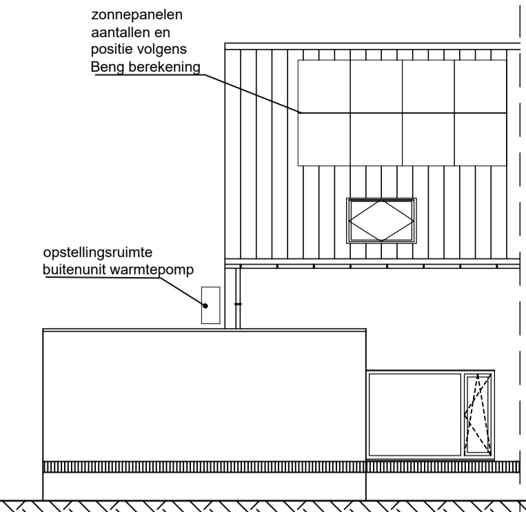
Achtergevel
