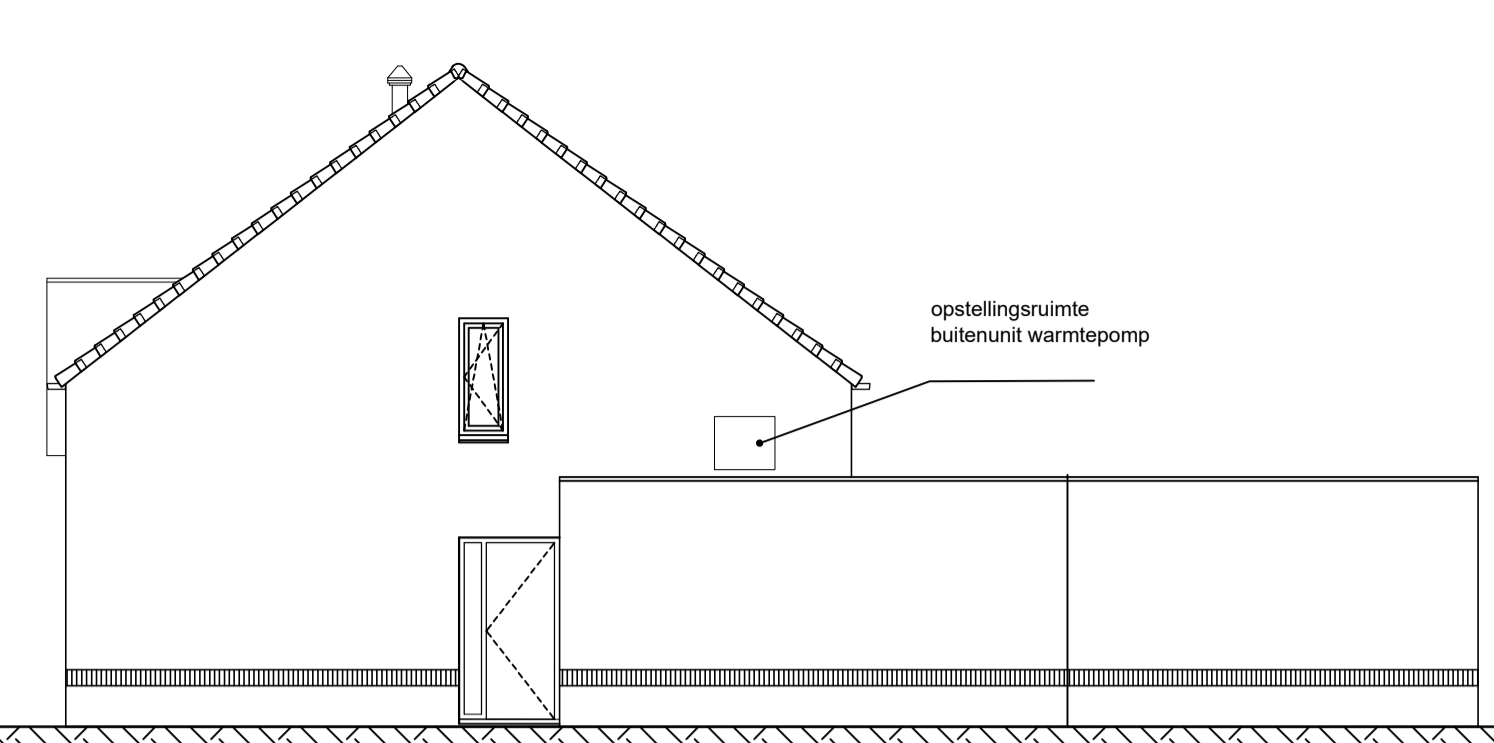
Rechter zijgevel
