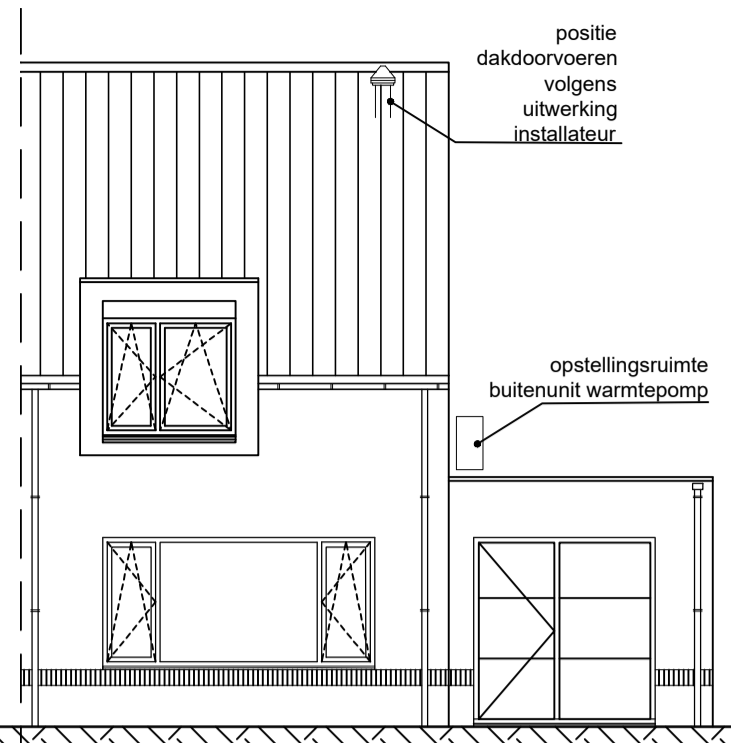
Voorgevel
