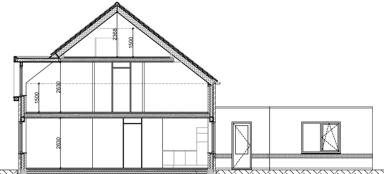
Doorsnede A - A Rechter zijgevel
