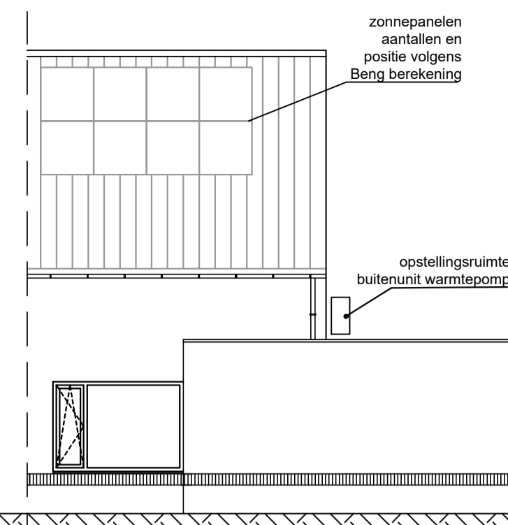
Achtergevel
