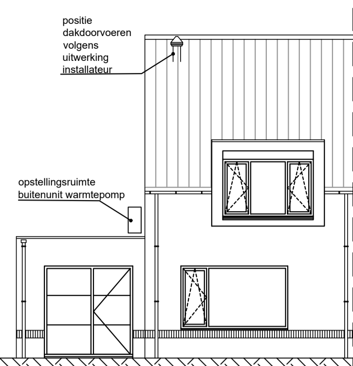
Voorgevel
